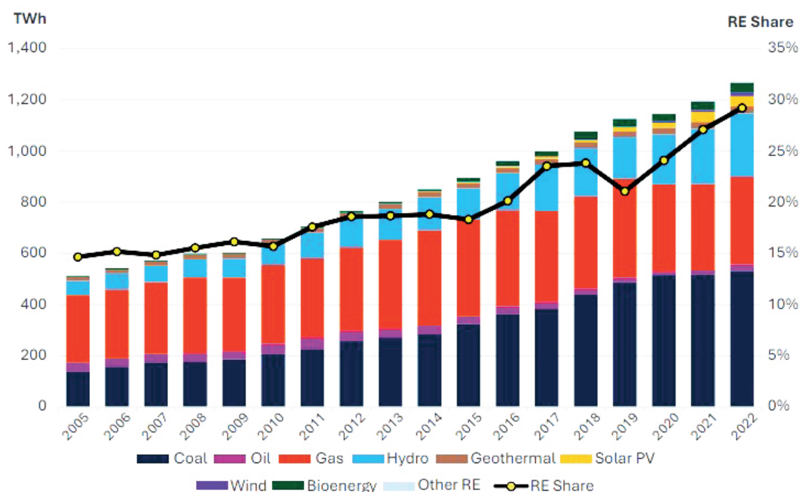
รูปที่ 1 แสดงการผลิตไฟฟ้ารวมของอาเซียน ปี 2005-2022
