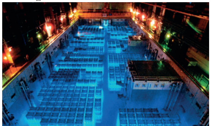
ตัวอย่างบ่อเก็บเชื้อเพลิงนิวเคลียร์ใช้แล้ว (Spent Fuel Pool)
