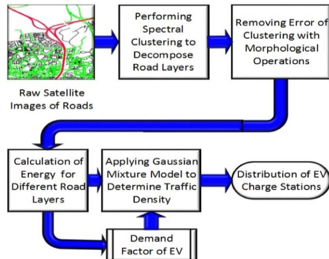
ภาพที่ 6 แผนภาพขั้นตอนการหาตำแหน่งสถานีอัดประจุด้วย Spectral Clustering และ Gaussian Mixture Model
