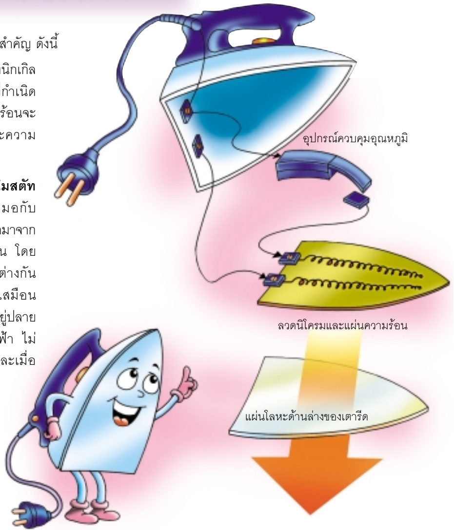
ส่วนประกอบของเตารีดไฟฟ้าแบบธรรมดา
