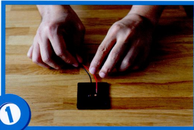
ต่อสายไฟเข้ากับขั้วที่อยู่บนหลังแผ่นเซลล์สุริยะ
