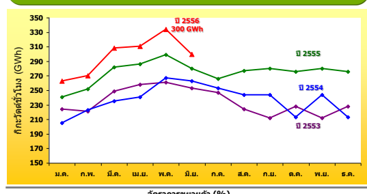
การใช้ไฟฟ้าอพาร์ทเมนต์และเกสต์เฮาส์ ปี 2553-2556 (ม.ย.)
