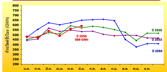
การใช้ไฟฟ้าอุตสาหกรรมอิเล็กทรอนิกส์ ปี 2553-2556 (มิ.ย.)
