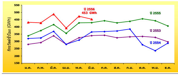
การใช้ไฟฟ้าอุตสาหกรรมการผลิตยานยนต์ ปี 2553-2556 (มิ.ย.)
