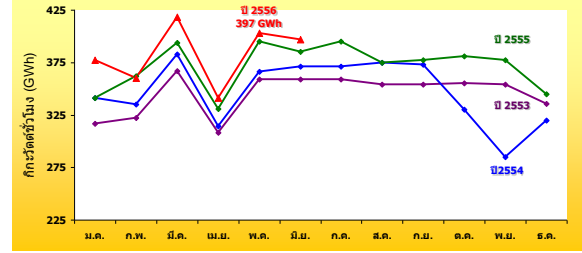
การใช้ไฟฟ้าอุตสาหกรรมพลาสติก ปี 2553-2556 (มิ.ย.)
