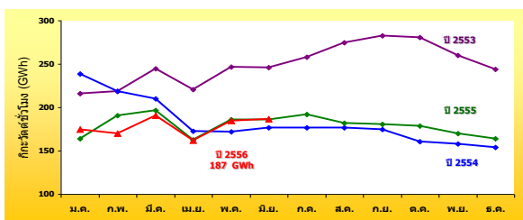
การใช้ไฟฟ้าอุตสาหกรรมเคมีภัณฑ์ ปี 2553-2556 (ม.ย.)
