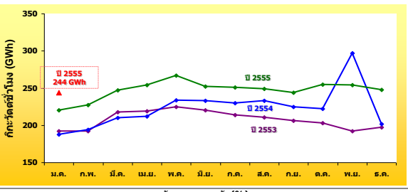
การใช้ไฟฟ้าร้านขายปลีก ปี 2553-2556 (ม.ค.)
