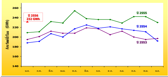
การใช้ไฟฟ้าอสังหาริมทรัพย์ ปี 2553-2556 (ม.ค.)
